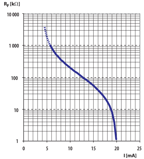
Stromausgang / Current output 4...20 mA
